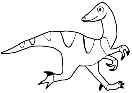
Compossognathus
