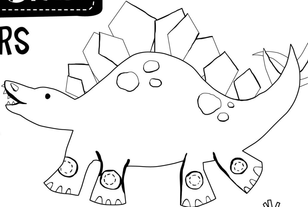
Stegosaurus
